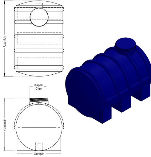
Teknik çizim
