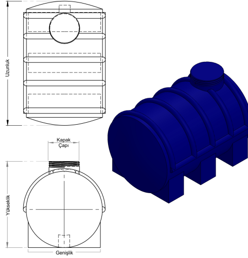
Teknik çizim
