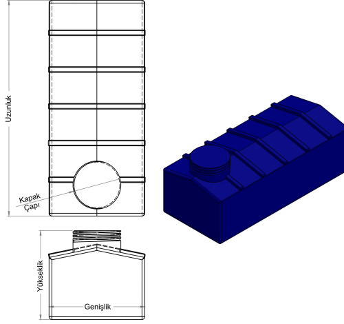
Teknik çizim
